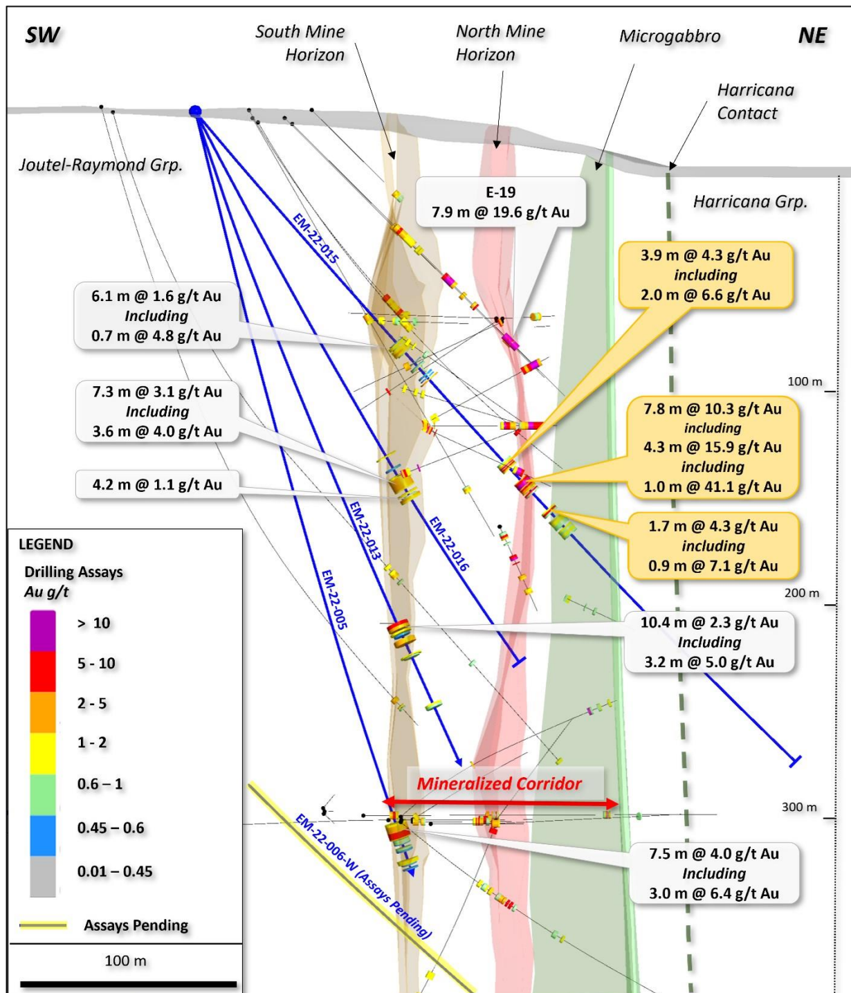
Figure 2: Section regardant vers le NW (épaisseur de 85m) montrant les nouveaux résultats (boîtes dorées) ainsi que les intersections historiques/précédemment annoncées (boîtes blanches) à l'intérieur d'horizons subparallèles bien définis.
