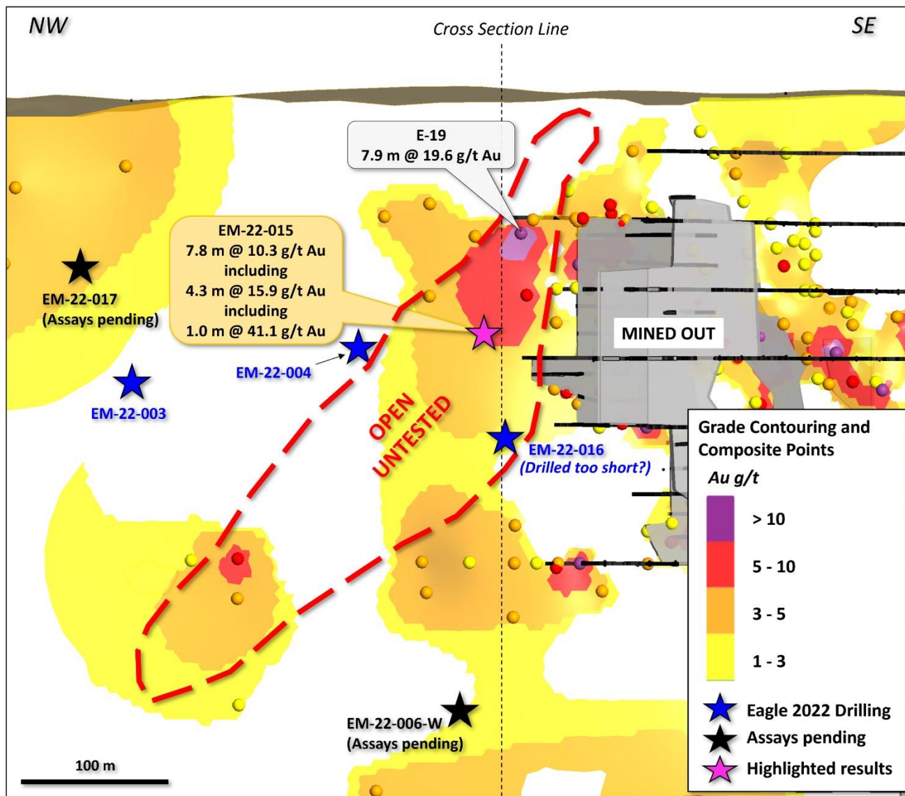
Figure 3: Longitudinale regardant vers le NE (épaisseur de 55m) montrant la localisation de l'intersection EM-22-015 (10,3 g/t Au sur 7,8 m) en relation avec les iso-contours des teneurs préexistantes du North Mine Horizon. Noté la surface ouverte et non testée de l'extension en plongé de la zone sous le forage E-19 (19,6 g/t Au sur 7,9m).
